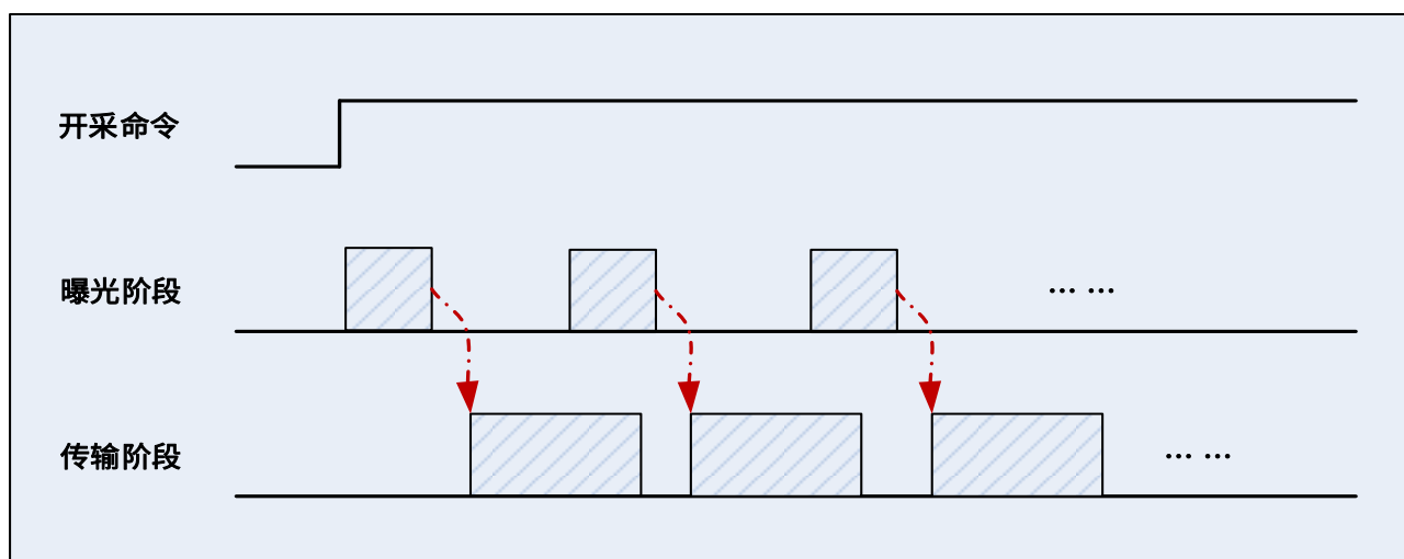
图 8-10 连续采集时序图
