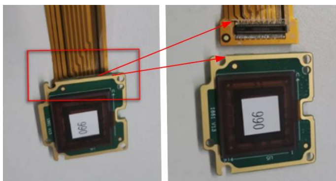
图 3-6 成像板连接器与 FPC 软线连接器处连接示意
