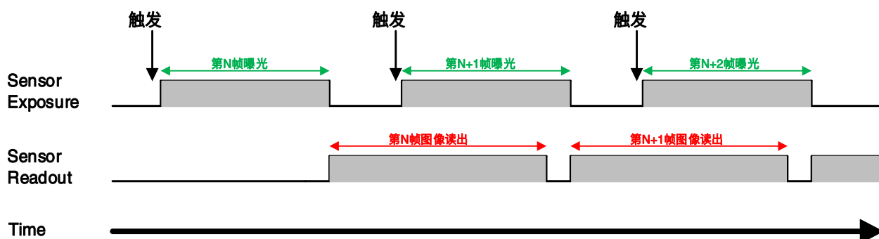
图 8-30 交叠曝光模式下触发采集曝光时序图
