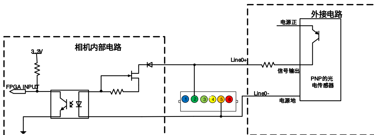
图 7-31 PNP 型光电传感器连接到光耦隔离输入电路
