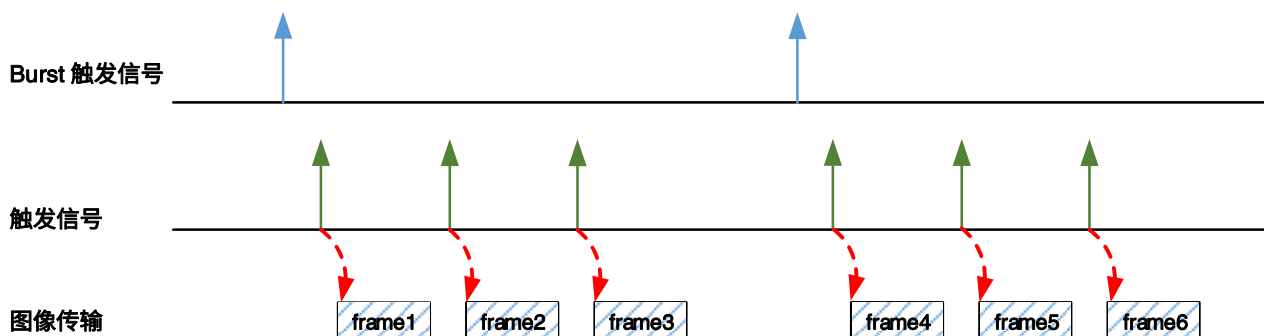
图 8-16 触发模式同时打开触发时序图
