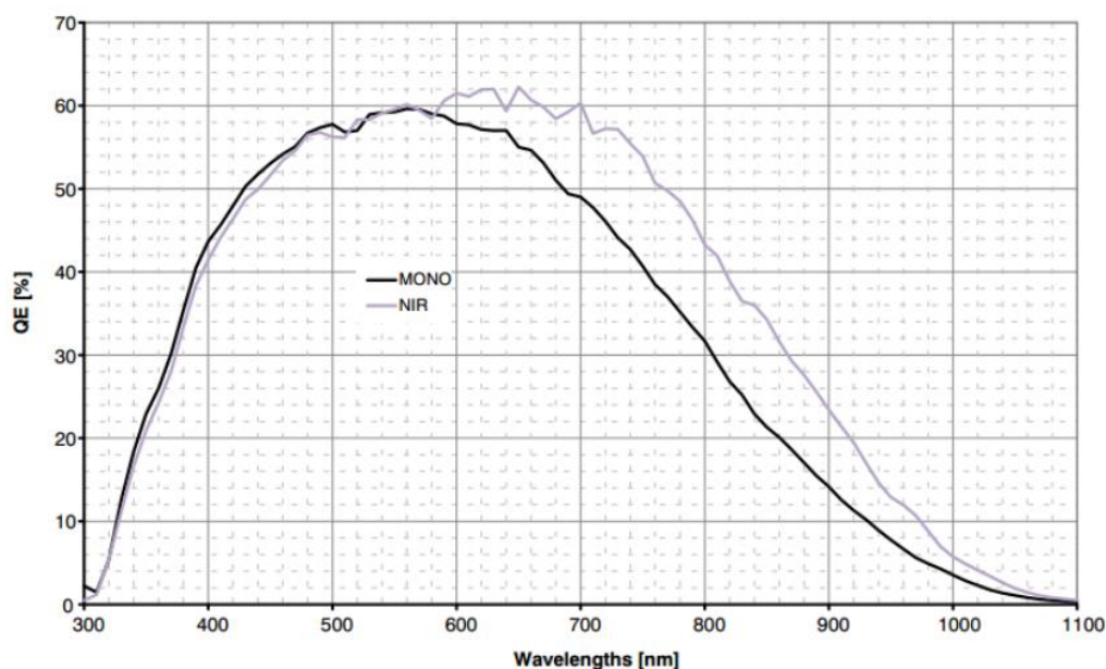
图 4-10 VEN-134-90U3M-D NIR SENSOR 响应曲线
