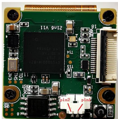
图 7-20 I/O 接口实物图
