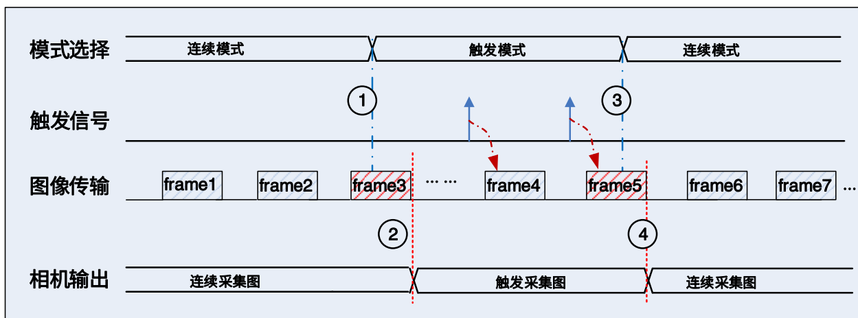
图 8-17 传输时切换触发模式
