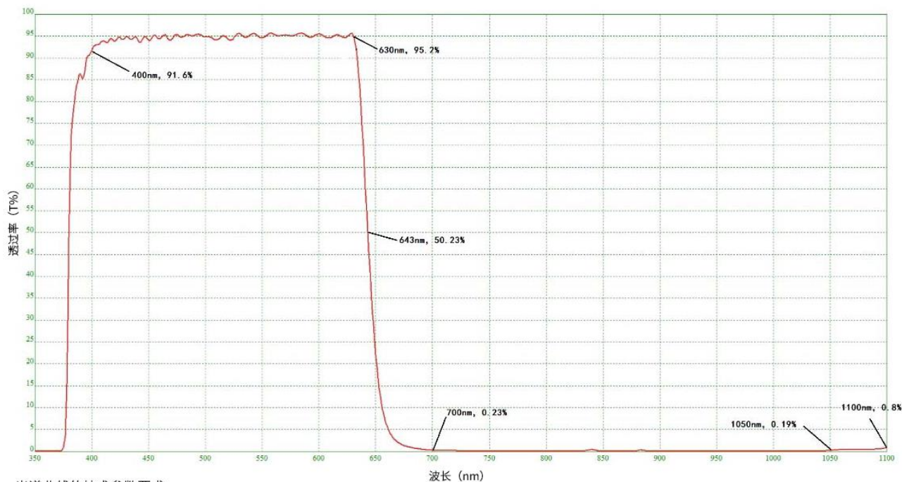
图 6-1 金星 USB3.0 彩色相机滤色片透过率曲线
