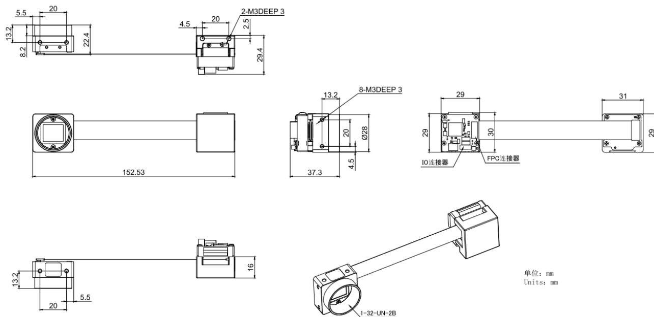
图 5-15 分体式垂直 FPC 相机尺寸
