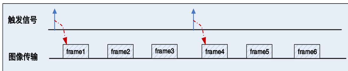
图 8-15 帧高速连拍开始触发时序图
