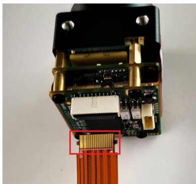
图 3-20 FPC 软线连接 FPC 座
