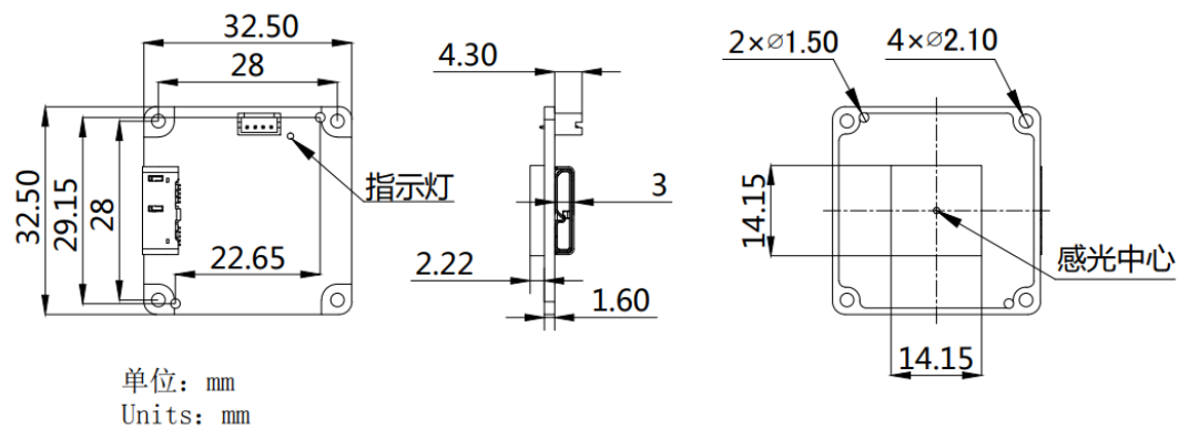
图 5-3 VEN-161-61U3M/C-M06 机械尺寸图
