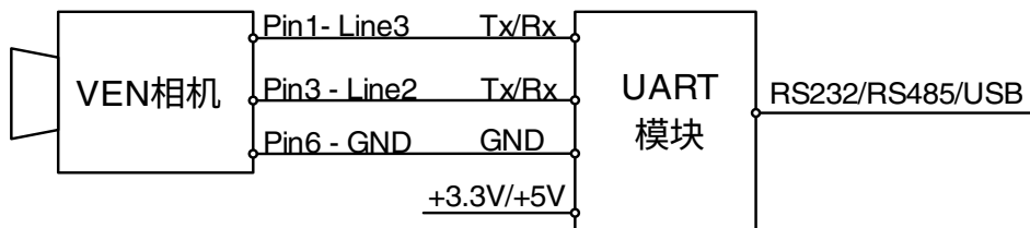
图 8-70 相机和外部串口设备的接线图
