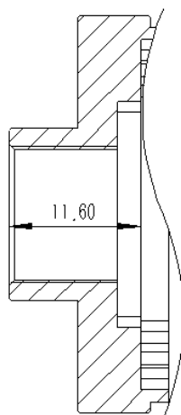
图 5-19 金星 USB3.0 相机 S 口光学接口（除一体式 FPC 相机）
