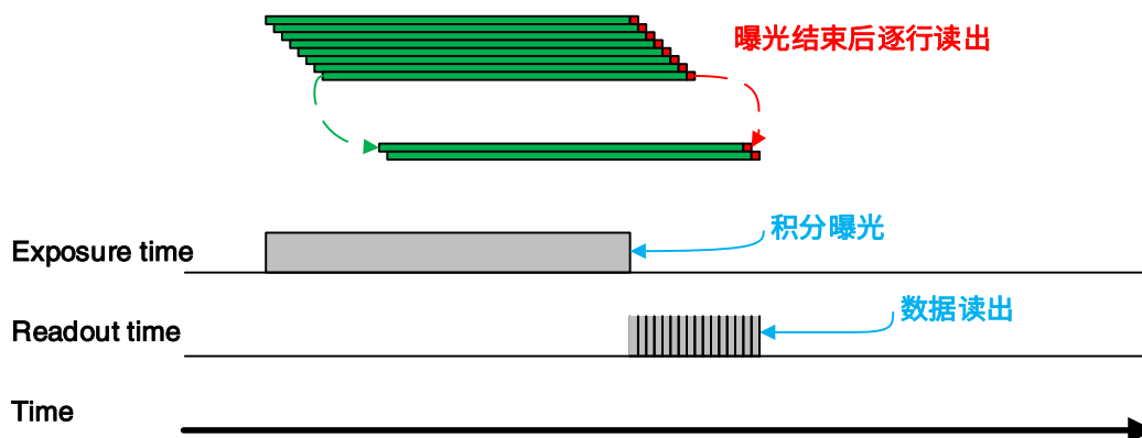
图 8-25 逐行曝光模式
