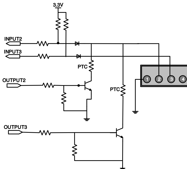
图 7-14 Line2/3 双向电路
