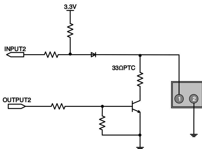
图 7-21 Line2（双向）电路
