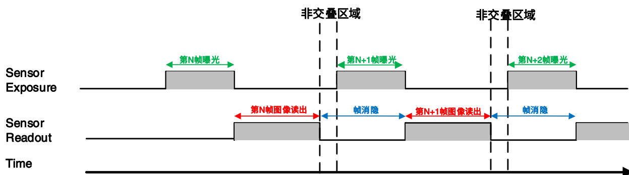
图 8-27 非交叠曝光模式下曝光时序图
