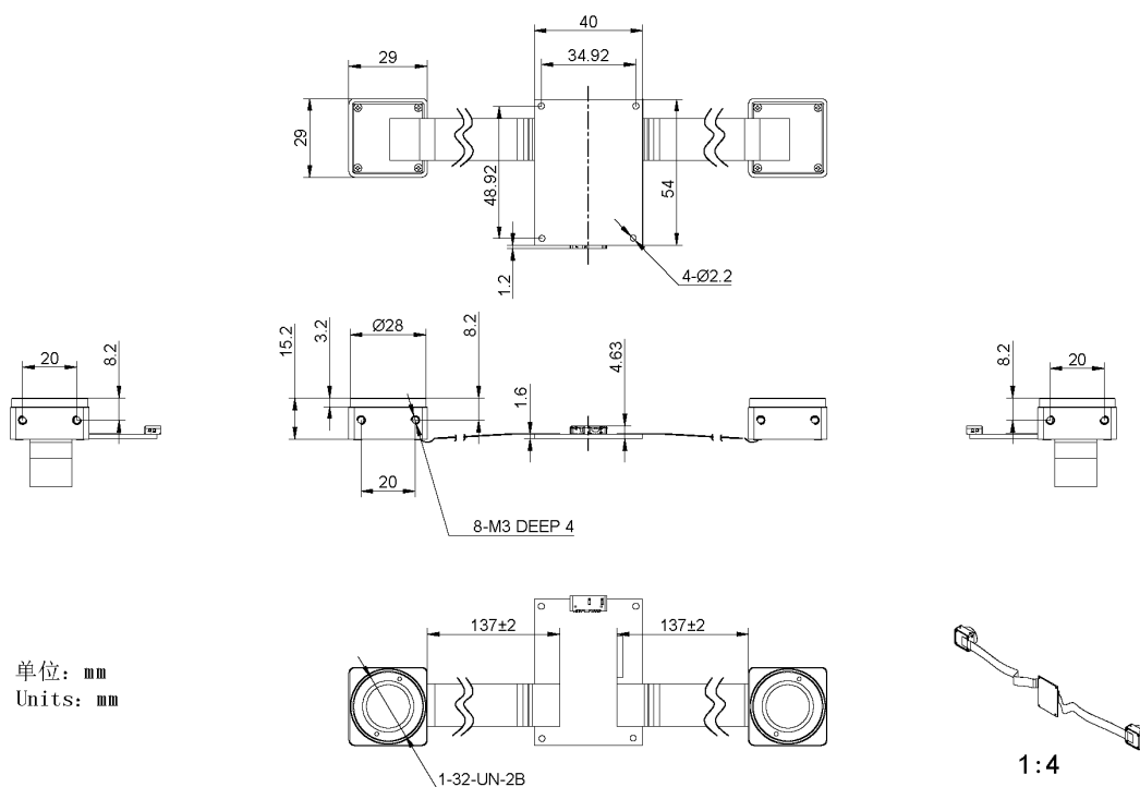
图 5-12 分体式 USB3 双目相机机械尺寸图 (CS-Mount)
