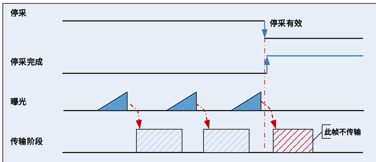
图 8-13 传输等待时停采时序图
