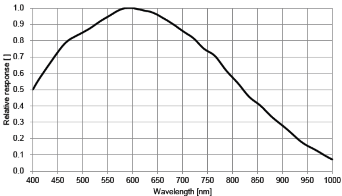
图 4-12 VEN-160-227U3M-FPC-(M00/M05) SENSOR 响应曲线
