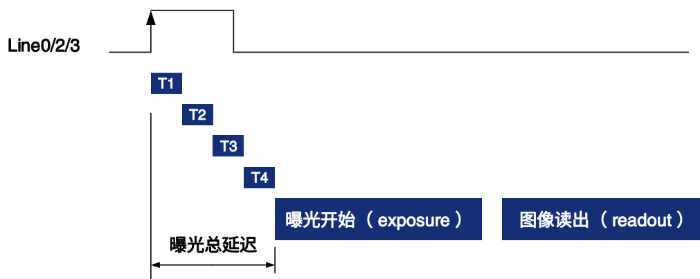
图 8-19 曝光延迟
