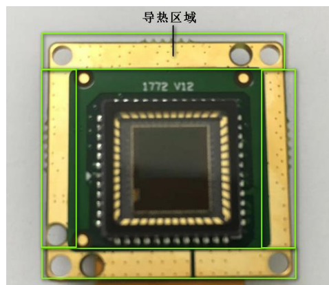
图 3-11 分体式双目相机成像板导热区域
