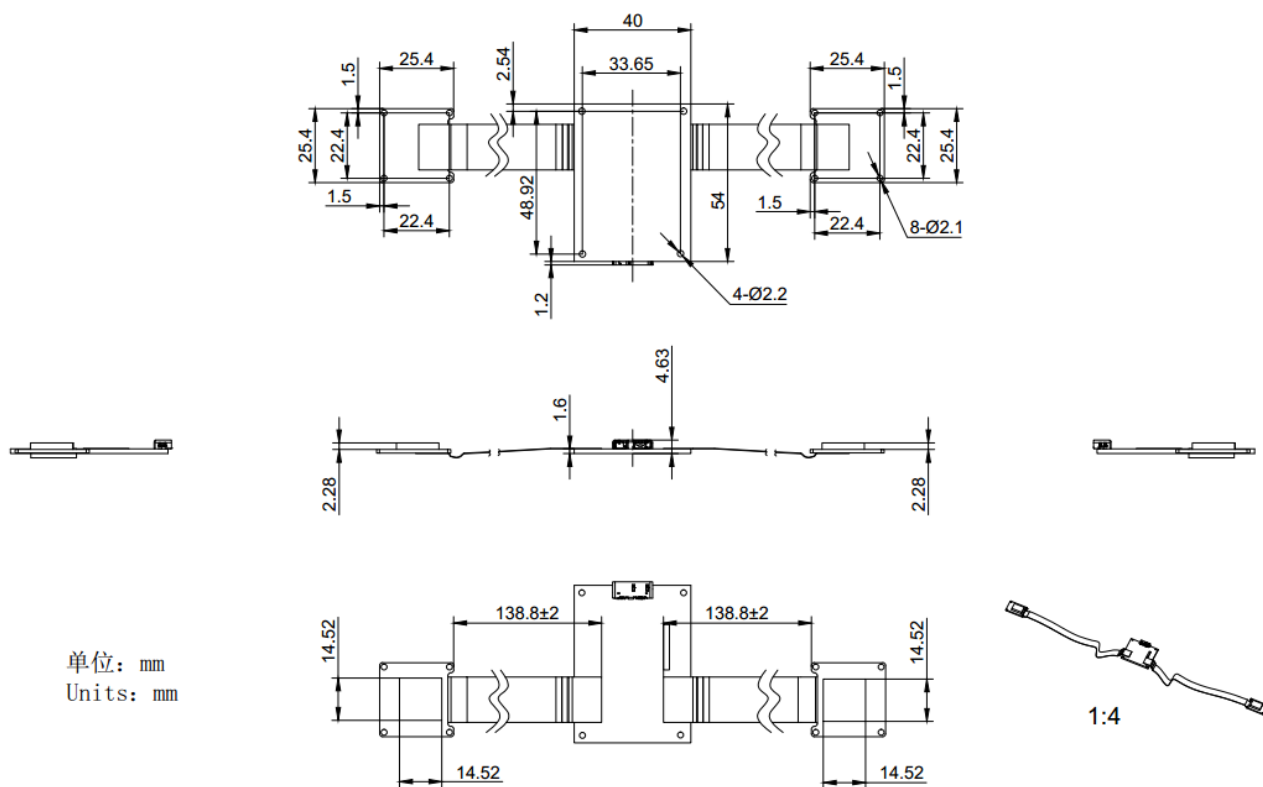
图 5-14 分体式 USB3 双目相机机械尺寸图 (No-Mount)
