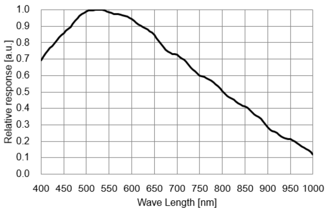
图 4-4 VEN-505-36U3M-(M01/M05/M06) SENSOR 响应曲线
