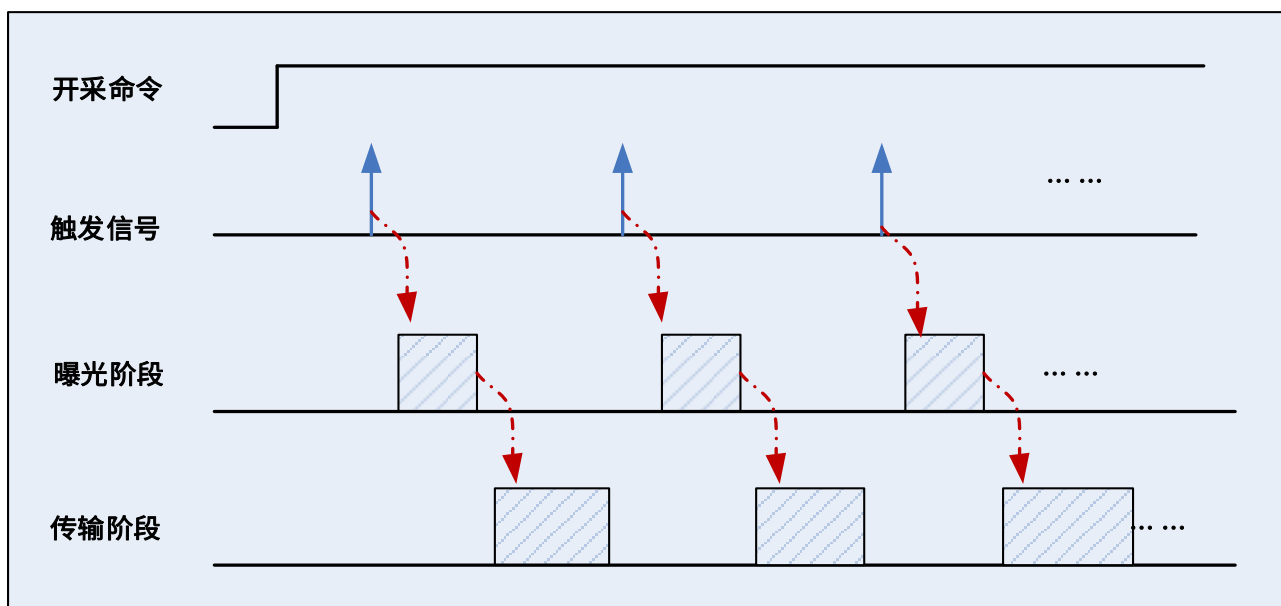
图 8-11 触发采集时序图
