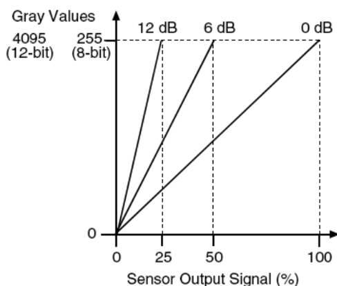
图 8-31 相机响应曲线
