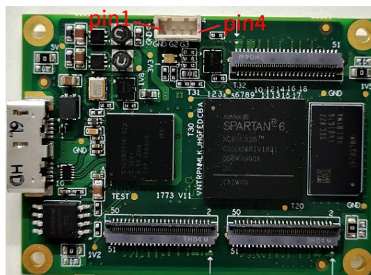
图 7-13 I/O 接口实物图
