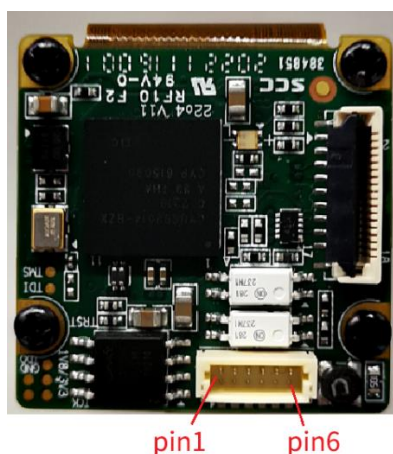
图 7-28 I/O 接口实物图
