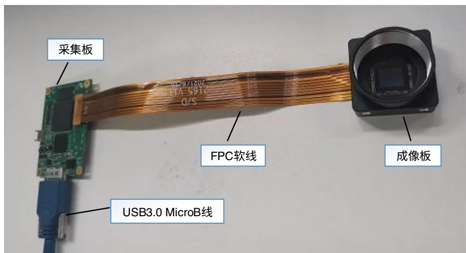
图 3-3 分体式单目相机组成和装配图（带 C-Mount）
