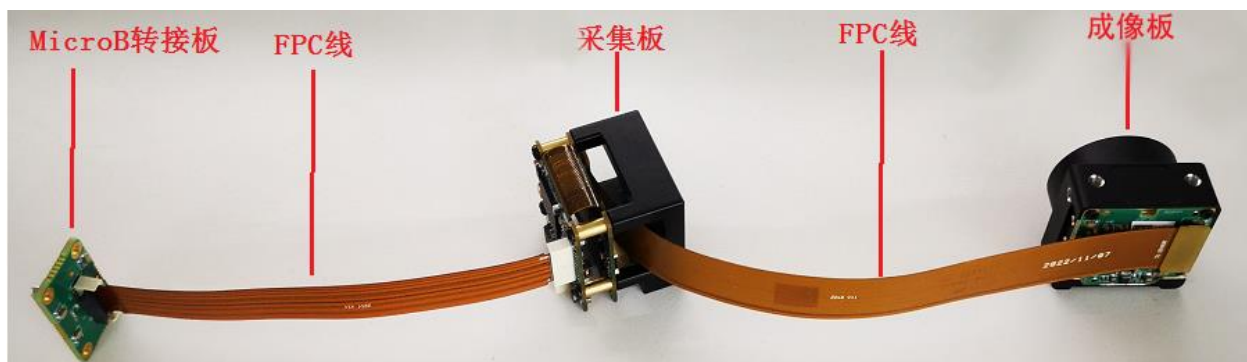
图 3-17 分体式垂直 FPC 相机组成和装配图
