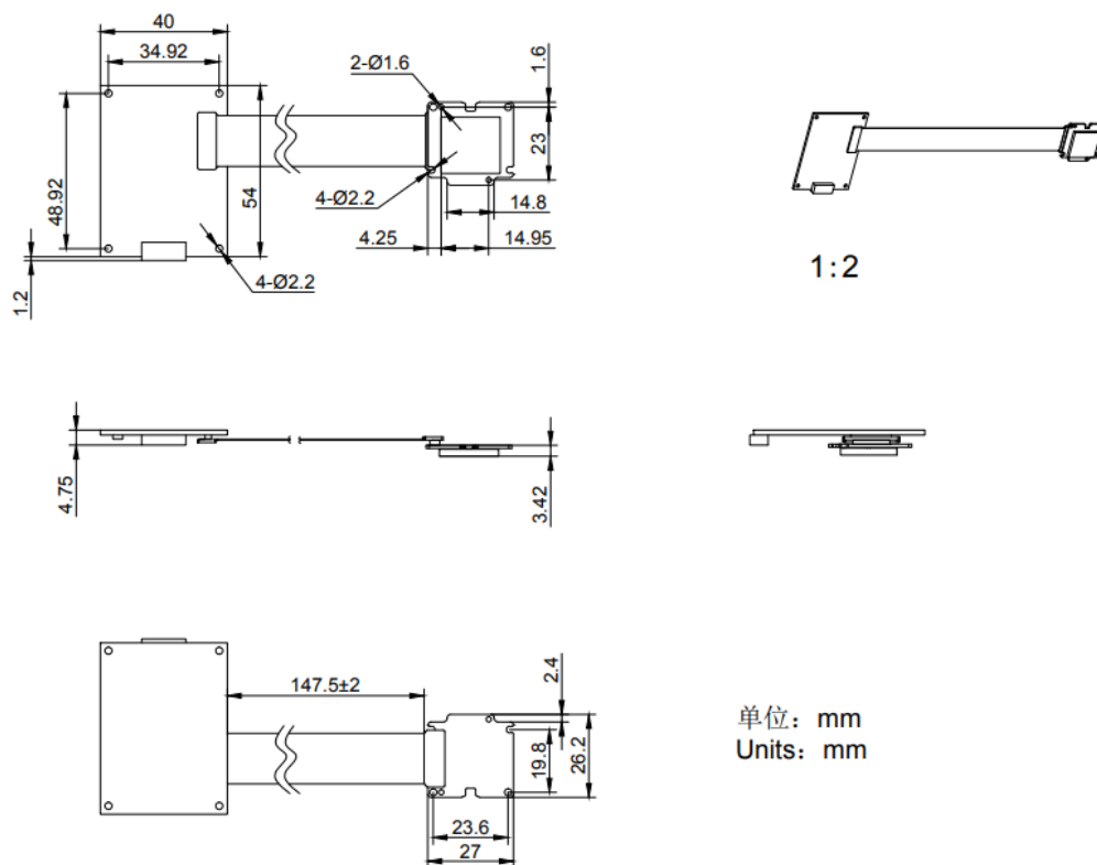
图 5-10 分体式 USB3 单目相机机械尺寸图 (No-Mount)
