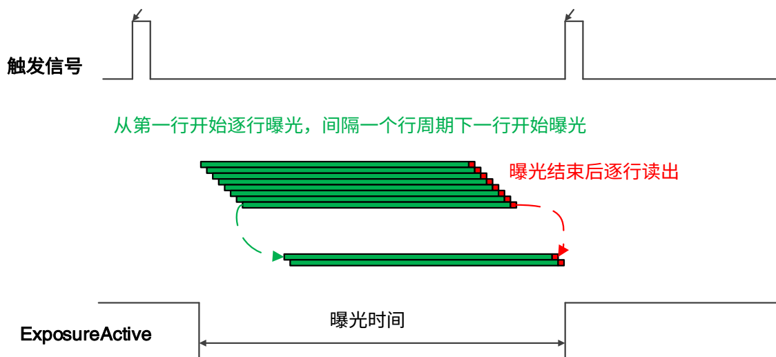
图 8-6 逐行曝光 ExposureActive 信号示意图
