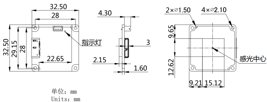
图 5-5 VEN-830-22U3M/C-M06 机械尺寸图
