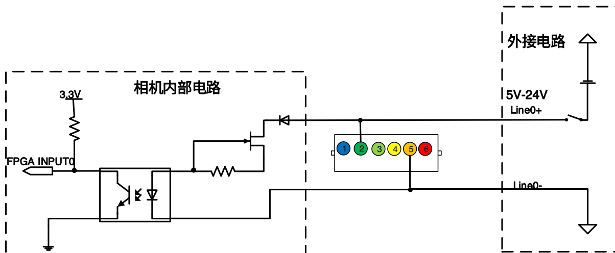
图 7-29 光耦隔离输入电路
