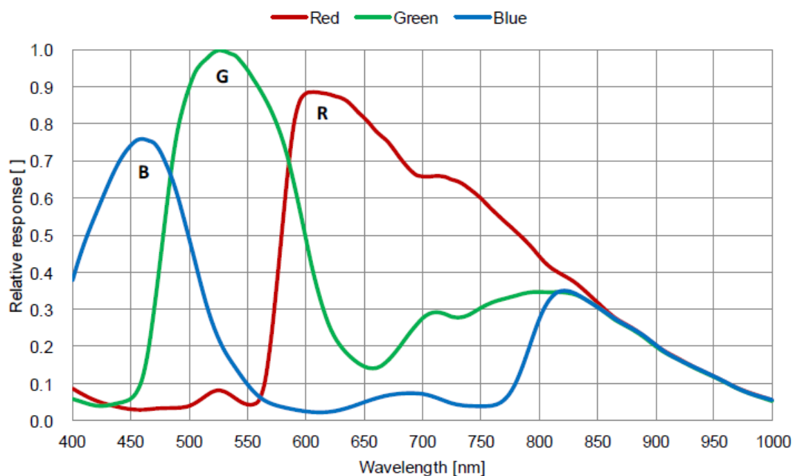
图 4-13 VEN-230-168U3C-FPC SENSOR 响应曲线
