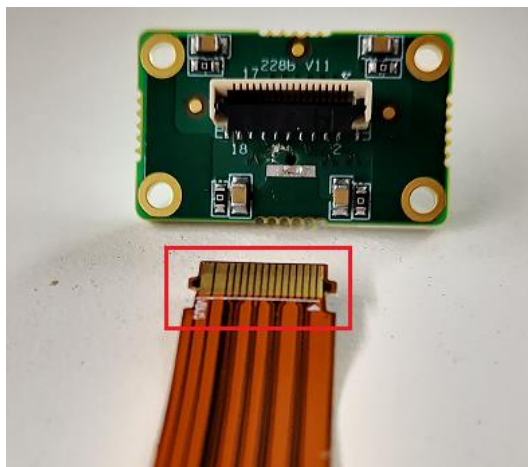
图 3-21 FPC 软线连接到 Micro-B 转接板
