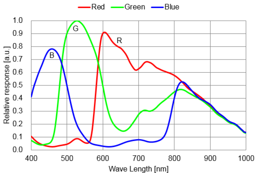
图 4-5 VEN-830-22U3C-(M01/M05/M06) SENSOR 响应曲线
