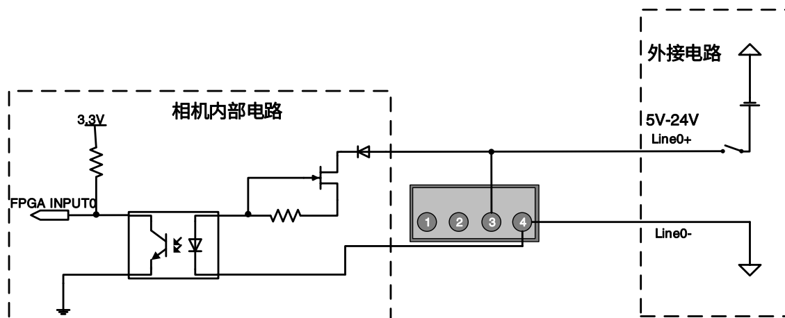
图 7-2 光耦隔离输入电路
