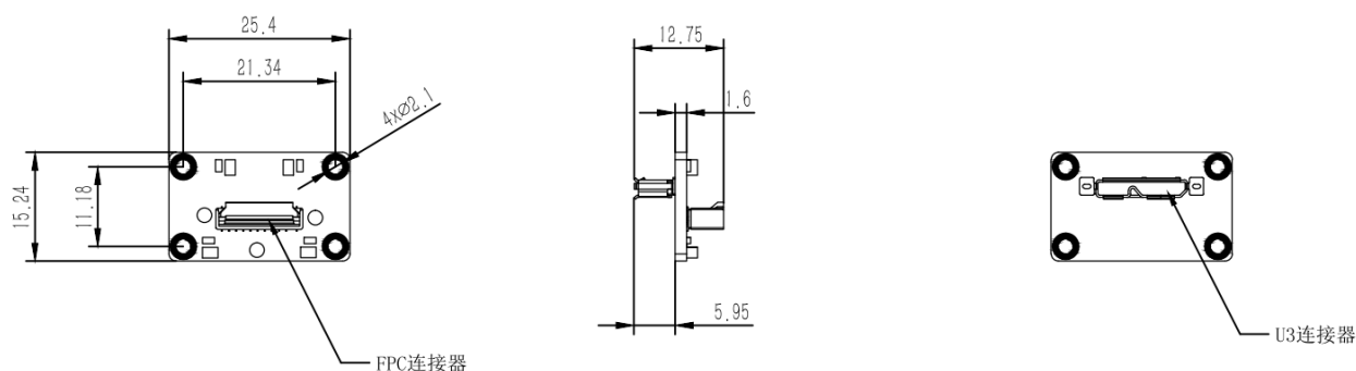
图 5-16 Micro-B 转接板尺寸
