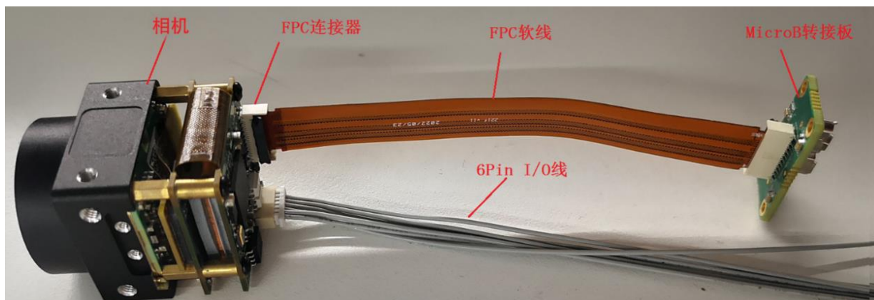
图 3-14 一体式垂直 FPC 相机组成和装配图
