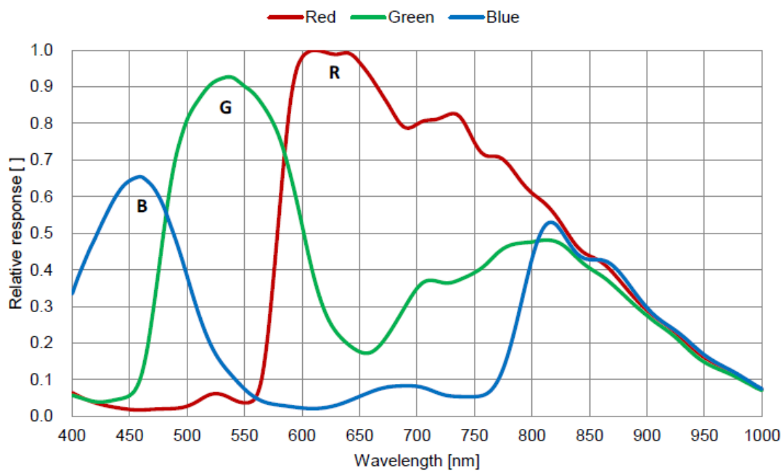
图 4-15 VEN-301-125U3C-FPC SENSOR 响应曲线
