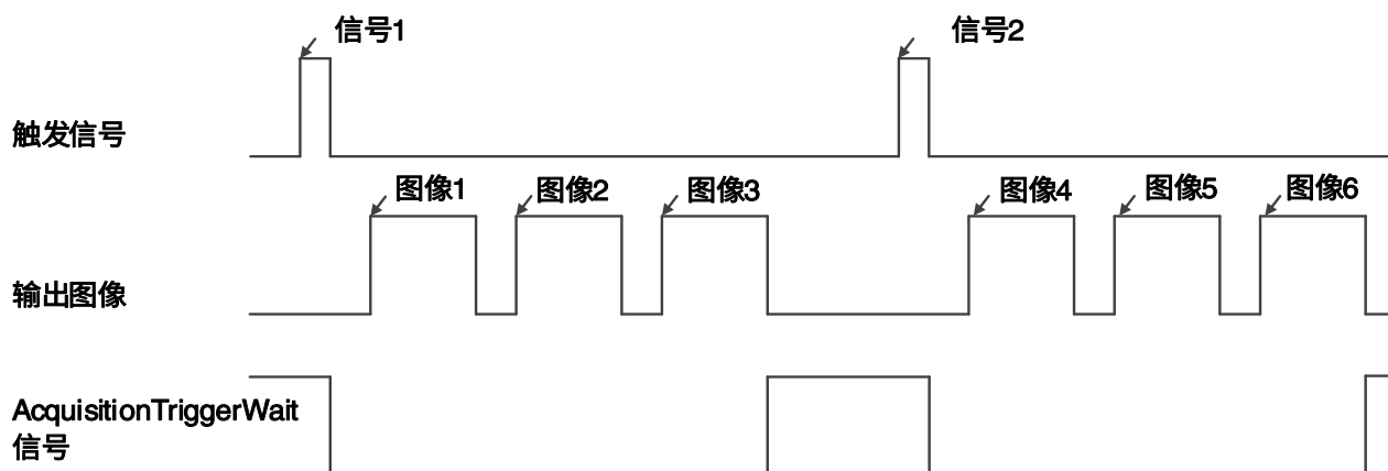
图 8-8 AcquisitionTriggerWait 信号示意图
