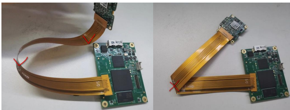
图 3-9 FPC 软线折叠
