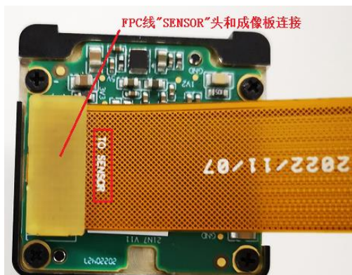
图 3-18 FPC 软线和成像板连接
