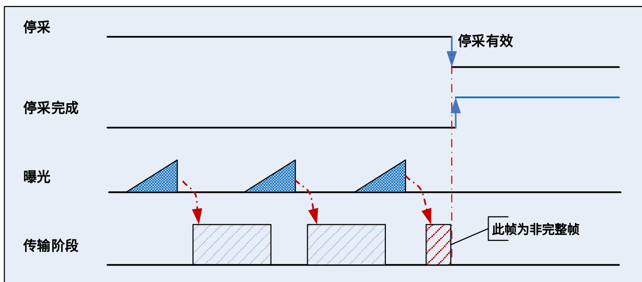
图 8-12 传输过程中停采时时序图
