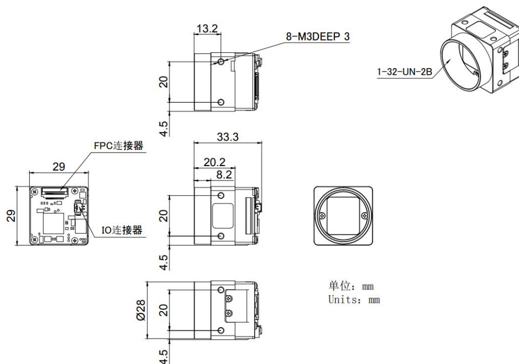
图 5-6 一体式水平 FPC 相机机械尺寸图 (C-Mount)
