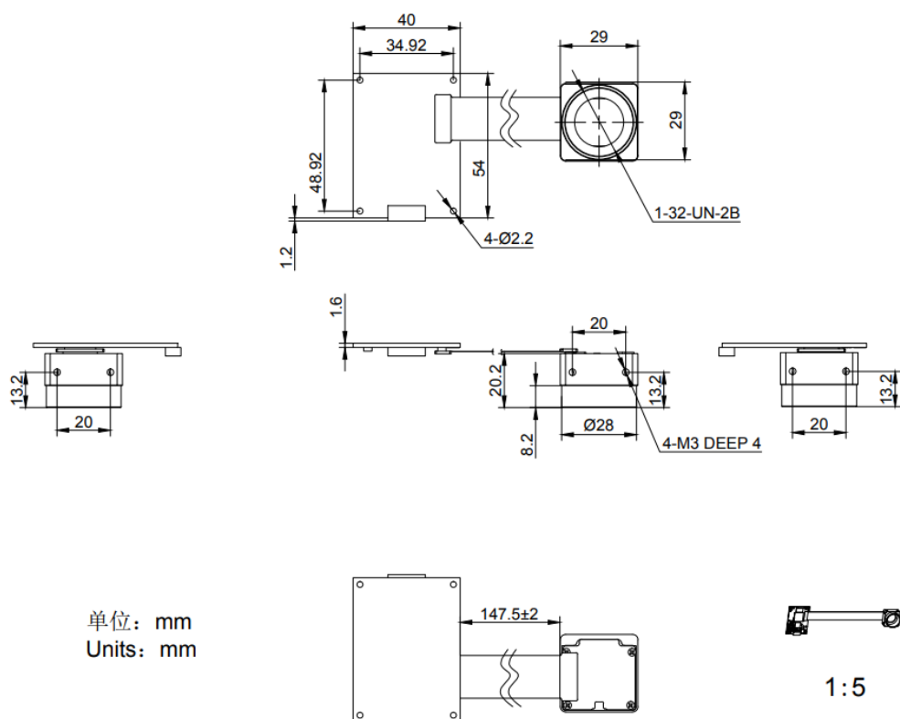
图 5-9 分体式 USB3 单目相机机械尺寸图 (C-Mount)
