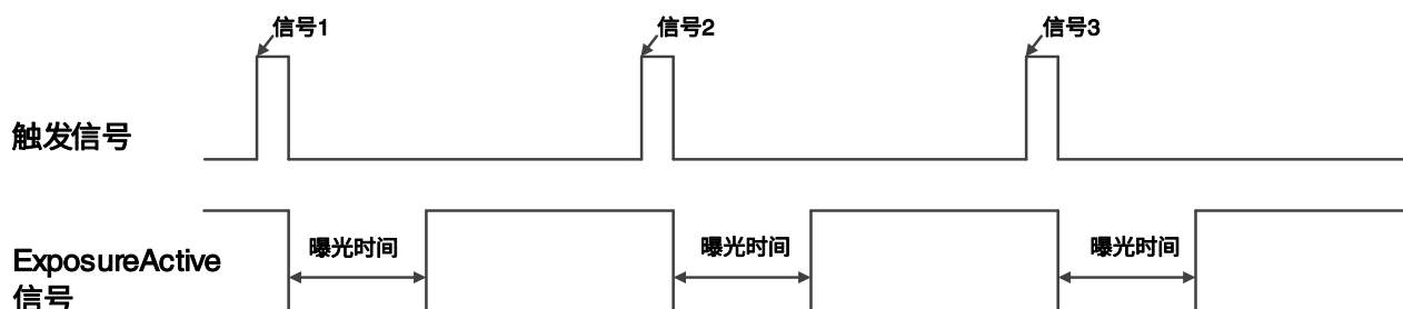
图 8-5 全局曝光模式 ExposureActive 信号示意图
