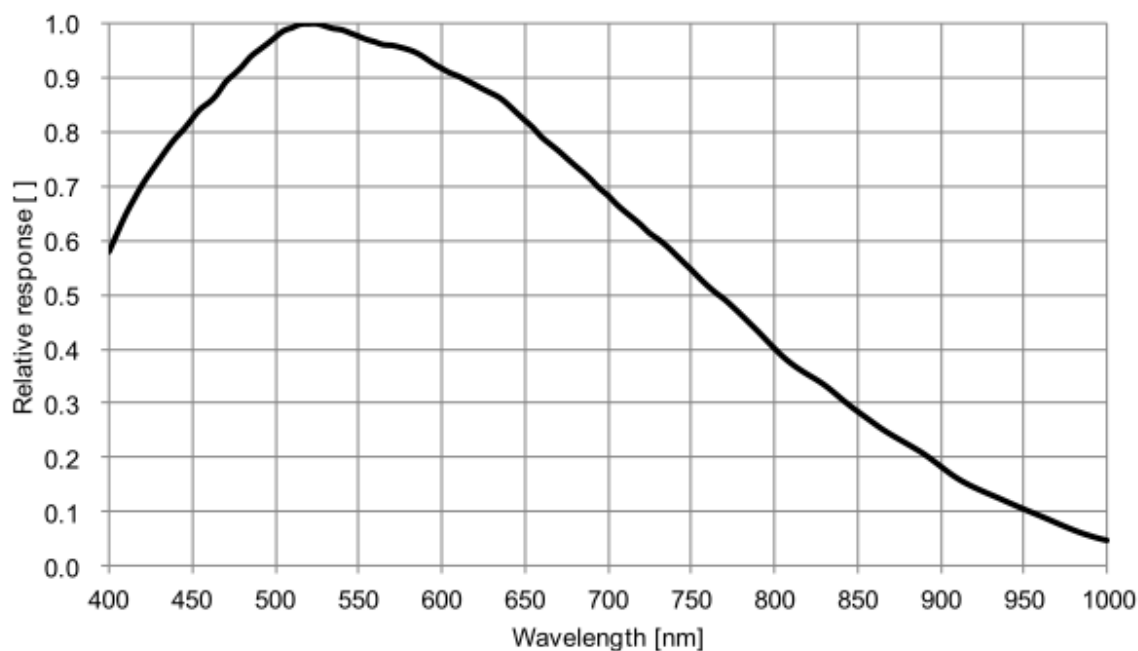
图 4-14 VEN-230-168U3M-FPC SENSOR 响应曲线
