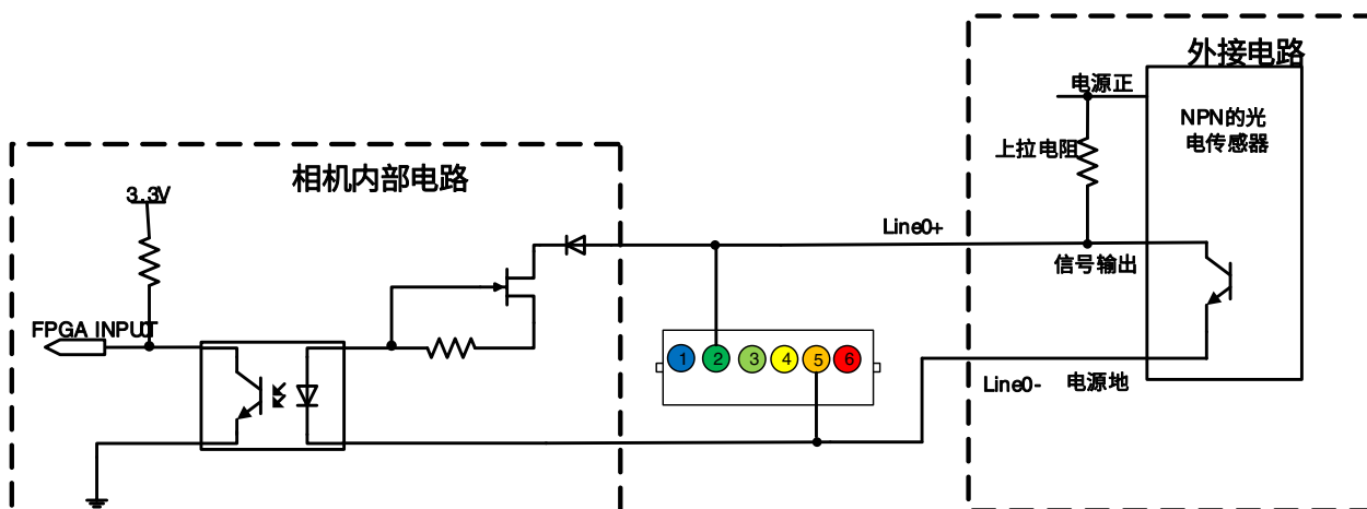
图 7-30 NPN 型光电传感器连接到光耦隔离输入电路
