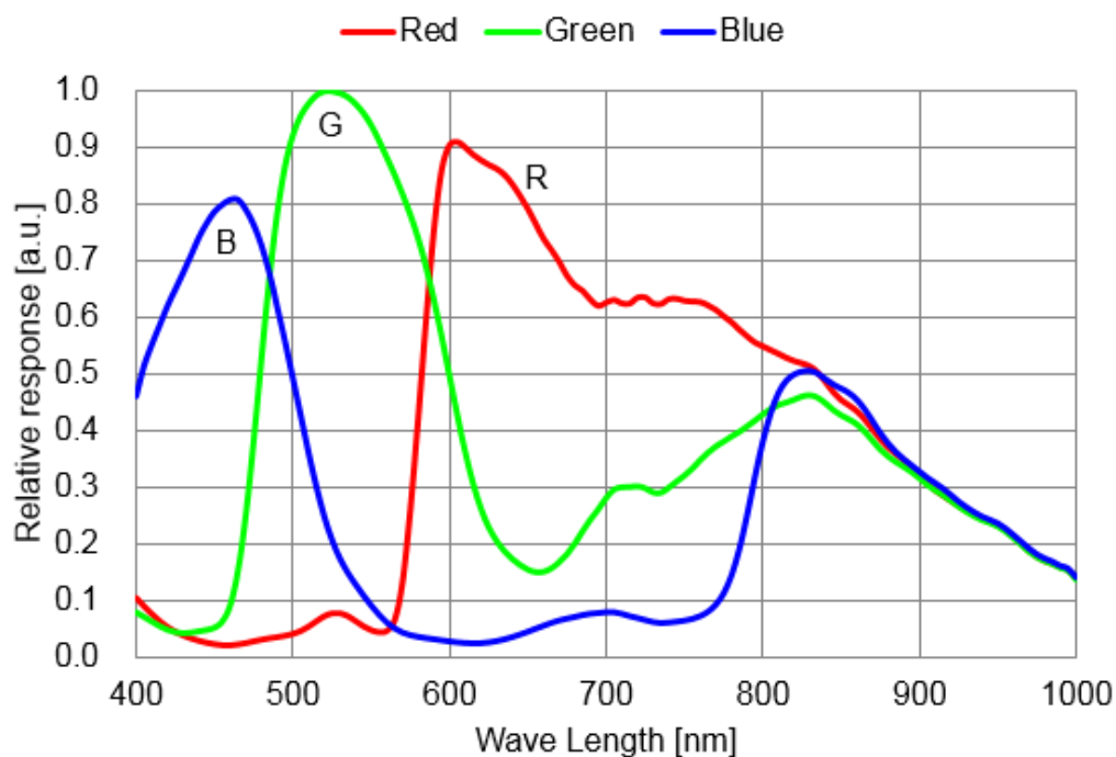
图 4-3 VEN-505-36U3C-(M01/M05/M06) SENSOR 响应曲线
