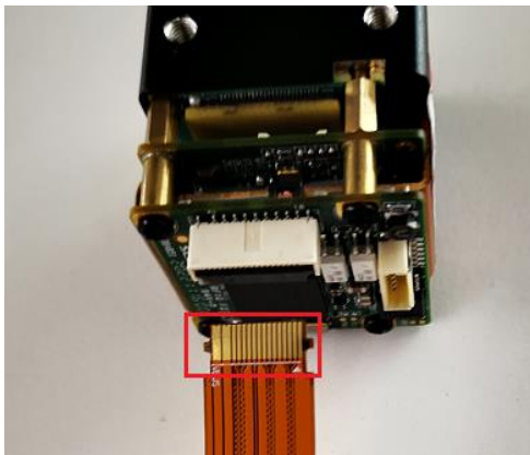
图 3-15 FPC 软线连接到相机
