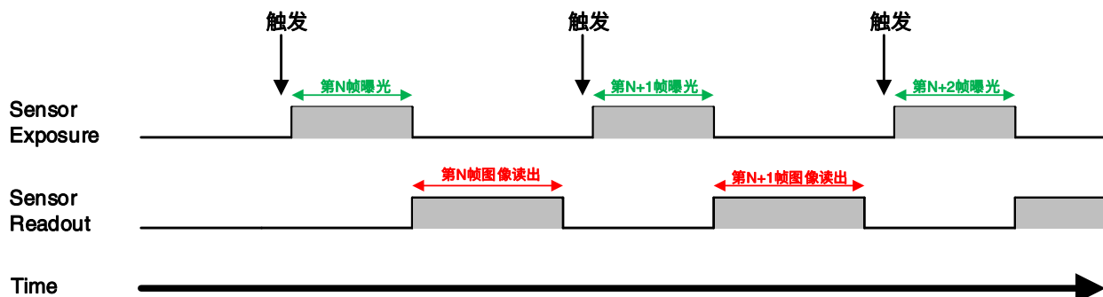
图 8-28 非交叠曝光模式下触发采集曝光时序图
