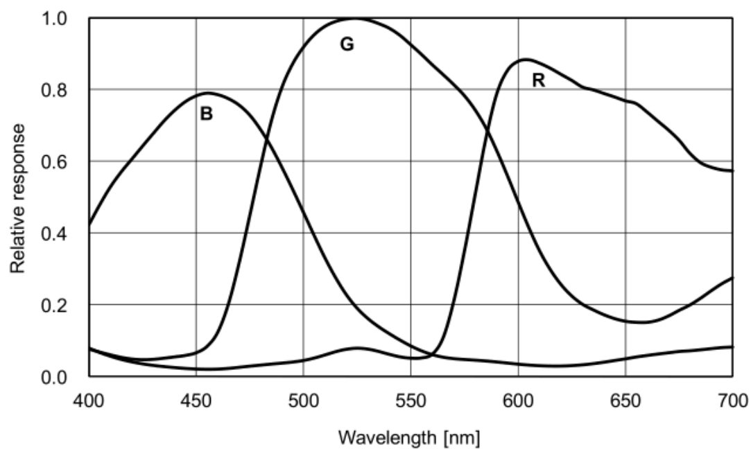
图 4-17 VEN-1220-32U3C-FPC-(M00/M05) SENSOR 响应曲线
