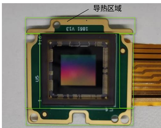
图 3-10 分体式单目相机成像板导热区域
