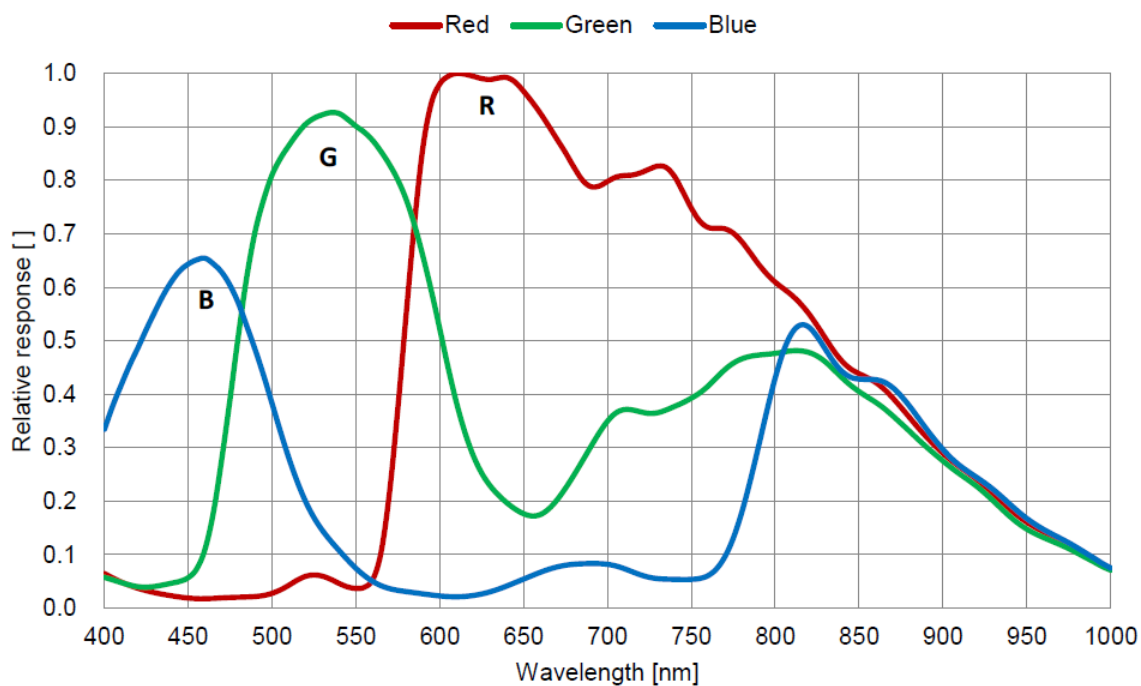
图 4-7 VEN-302-56U3C-S SENSOR 响应曲线
