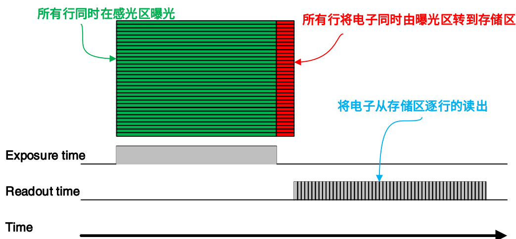
图 8-24 全局曝光模式
