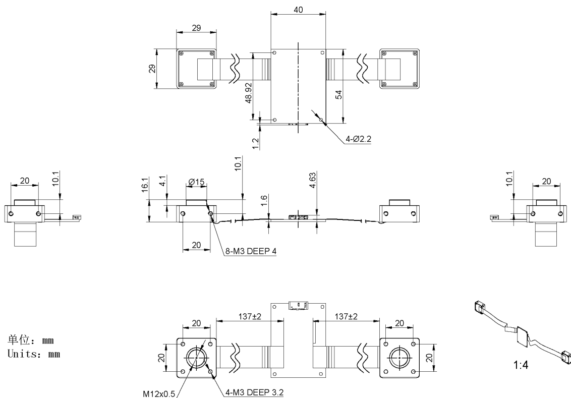
图 5-13 分体式 USB3 双目相机机械尺寸图 (S-Mount)
