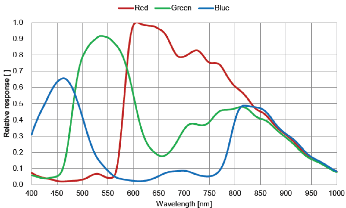
图 4-11 VEN-160-227U3C-FPC-(M00/M05) SENSOR 响应曲线
