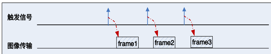
图 8-14 帧开始触发时序图
