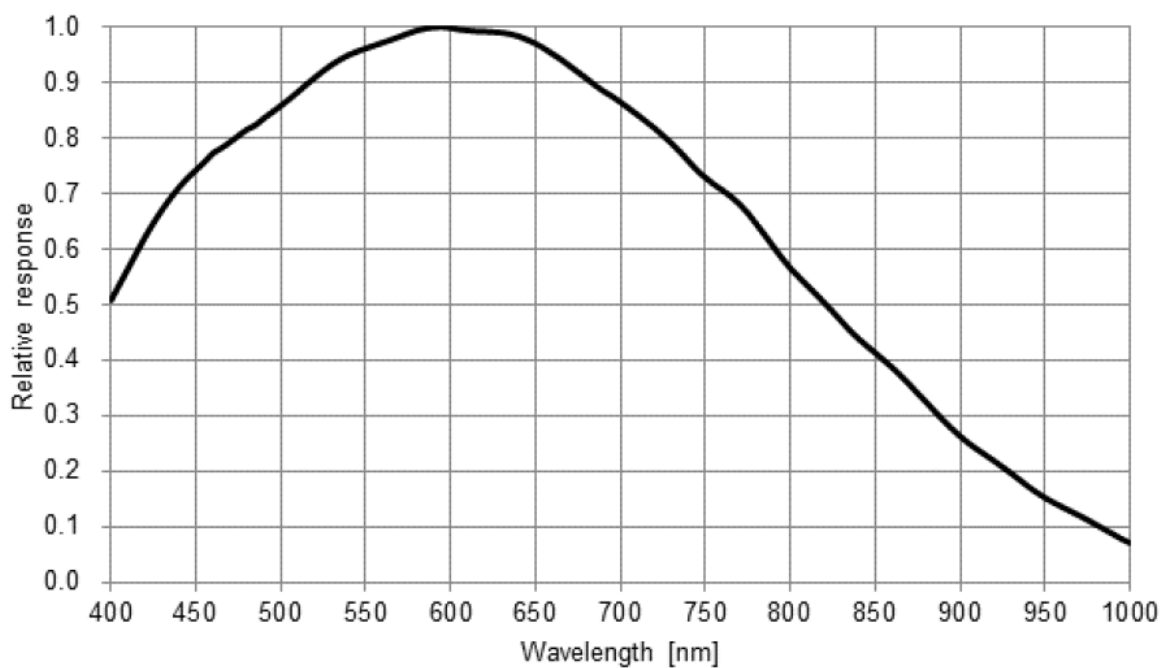
图 4-8 VEN-302-56U3M-S SENSOR 响应曲线
