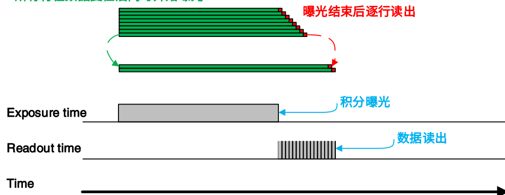
图 8-26 全局复位释放模式
