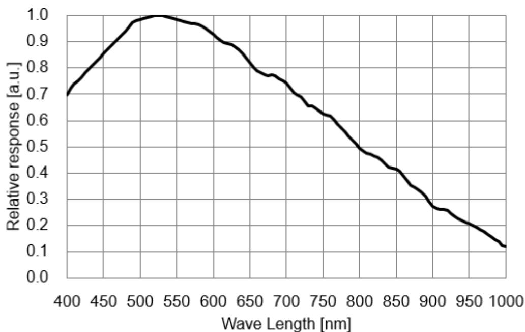
图 4-6 VEN-830-22U3M-(M01/M05/M06) SENSOR 响应曲线
