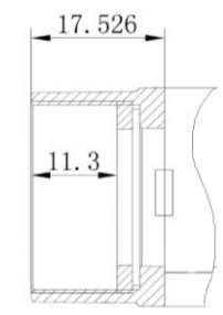
图 5-17 金星 USB3.0 相机 C 口光学接口
