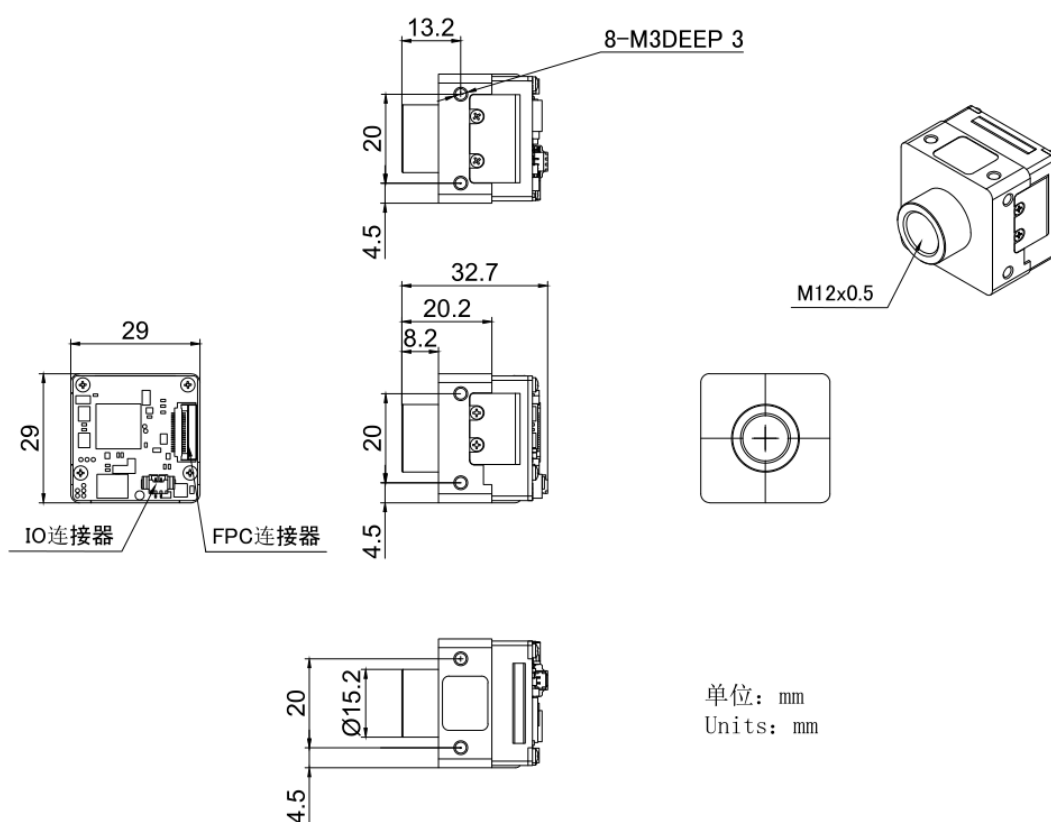
图 5-7 一体式水平 FPC 相机机械尺寸图 (S-Mount)
