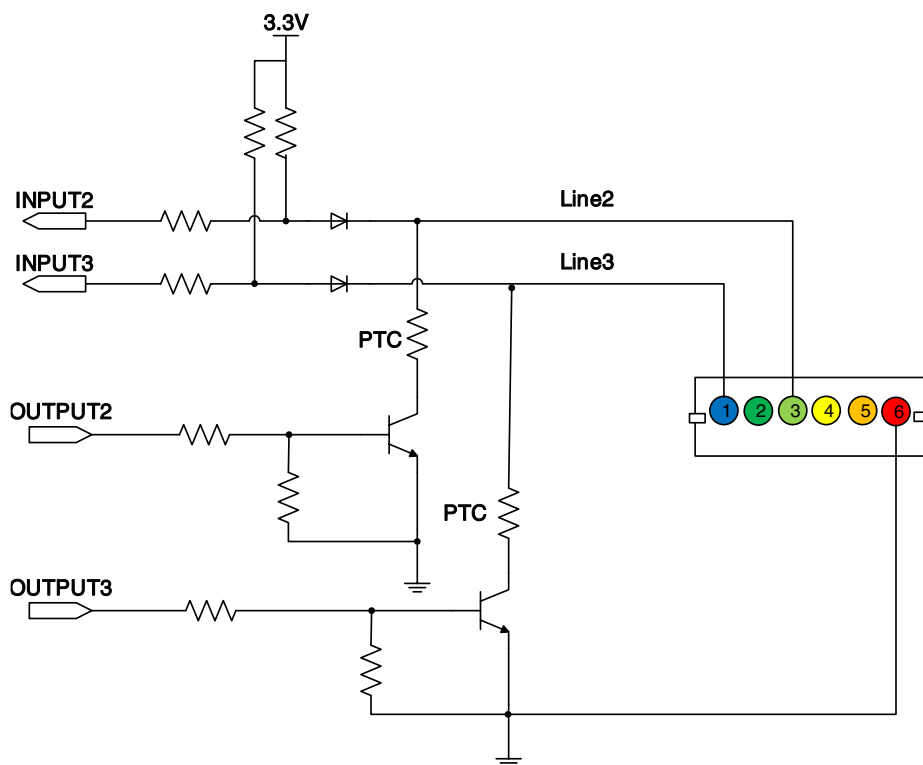
图 7-35 Line2/3 (双向) 电路
