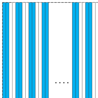
图 8-48 彩色相机水平像素抽样原理
