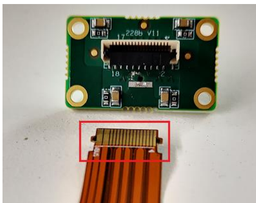
图 3-16 FPC 软线连接到 Micro-B 转接板
