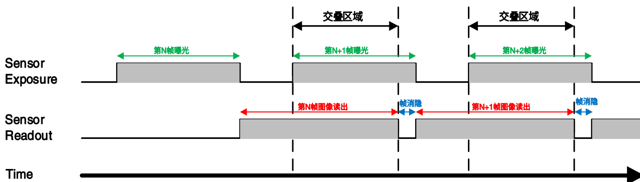
图 8-29 交叠曝光模式下曝光时序图
