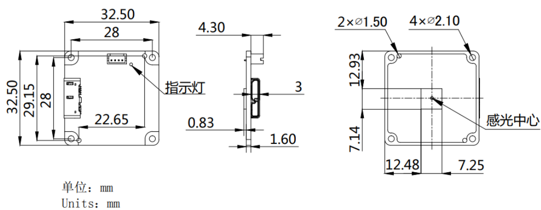
图 5-4 VEN-505-36U3M/C-M06 机械尺寸图
