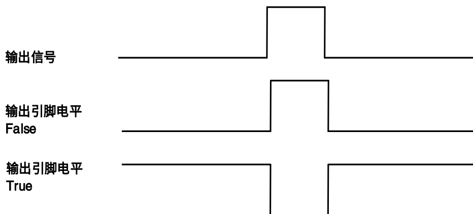
图 8-9 设置输出引脚反向
