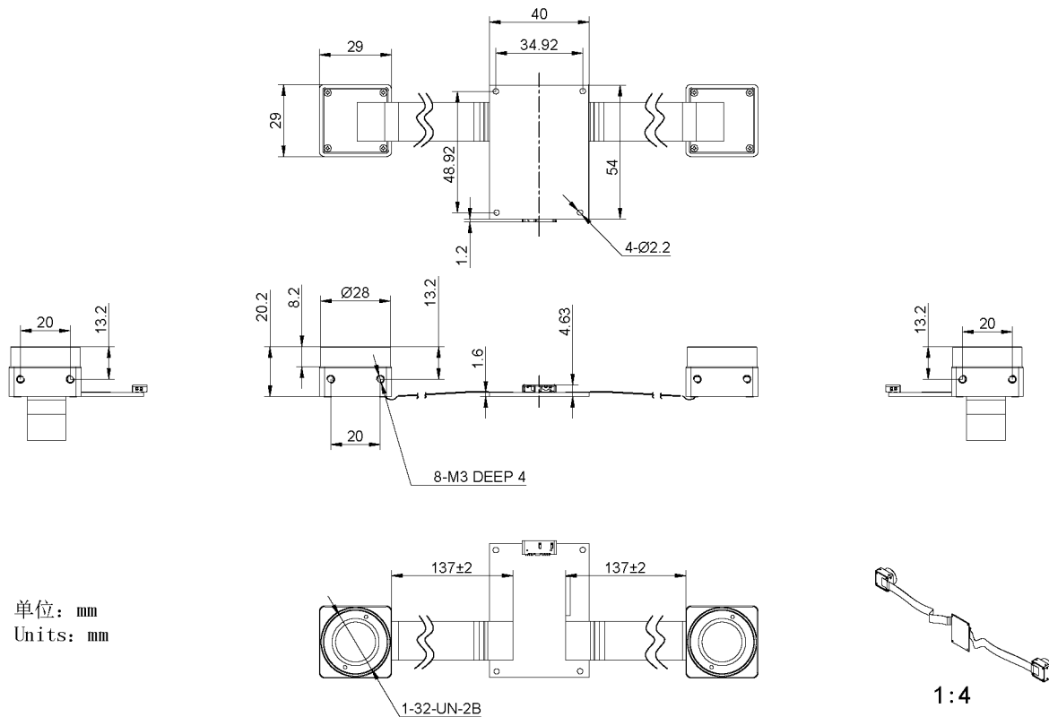
图 5-11 分体式 USB3 双目相机机械尺寸图 (C-Mount)
