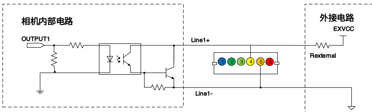
图 7-33 光耦隔离输出电路
