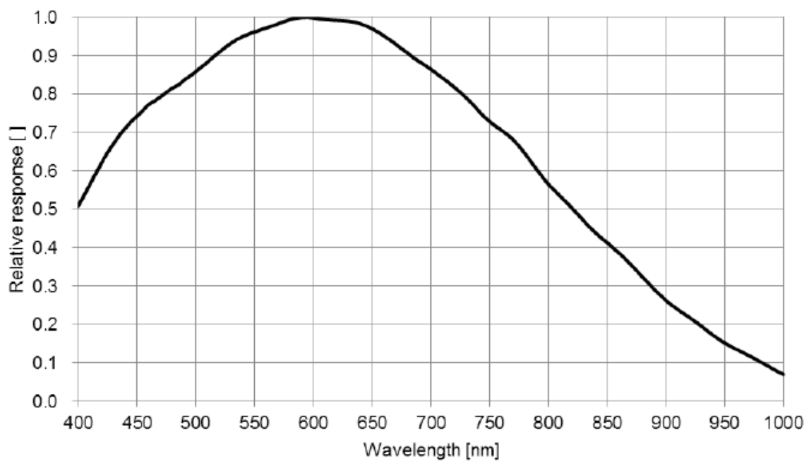
图 4-16 VEN-301-125U3M-FPC SENSOR 响应曲线
