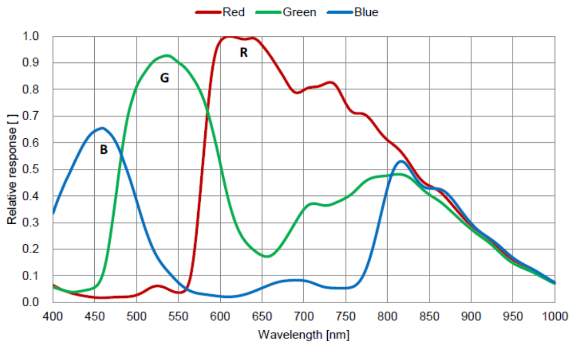
图 4-19 VE2S-301-125U3C-S (J150) SENSOR 响应曲线
