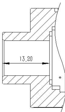
图 5-20 一体式 FPC 相机 S 口光学接口
