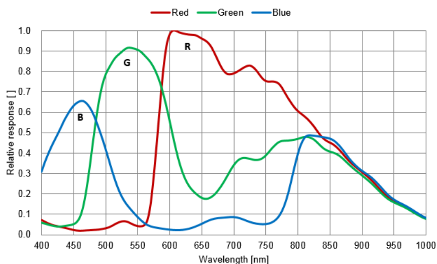
图 4-1 VEN-161-61U3C-(M01/M05/M06) SENSOR 响应曲线
