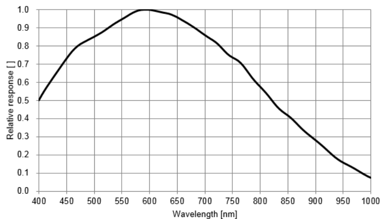
图 4-2 VEN-161-61U3M-(M01/M05/M06) SENSOR 响应曲线
