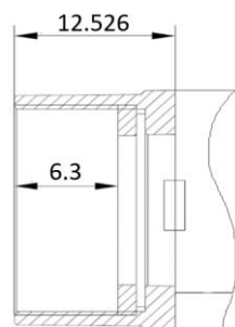
图 5-18 金星 USB3.0 相机 CS 口光学接口
