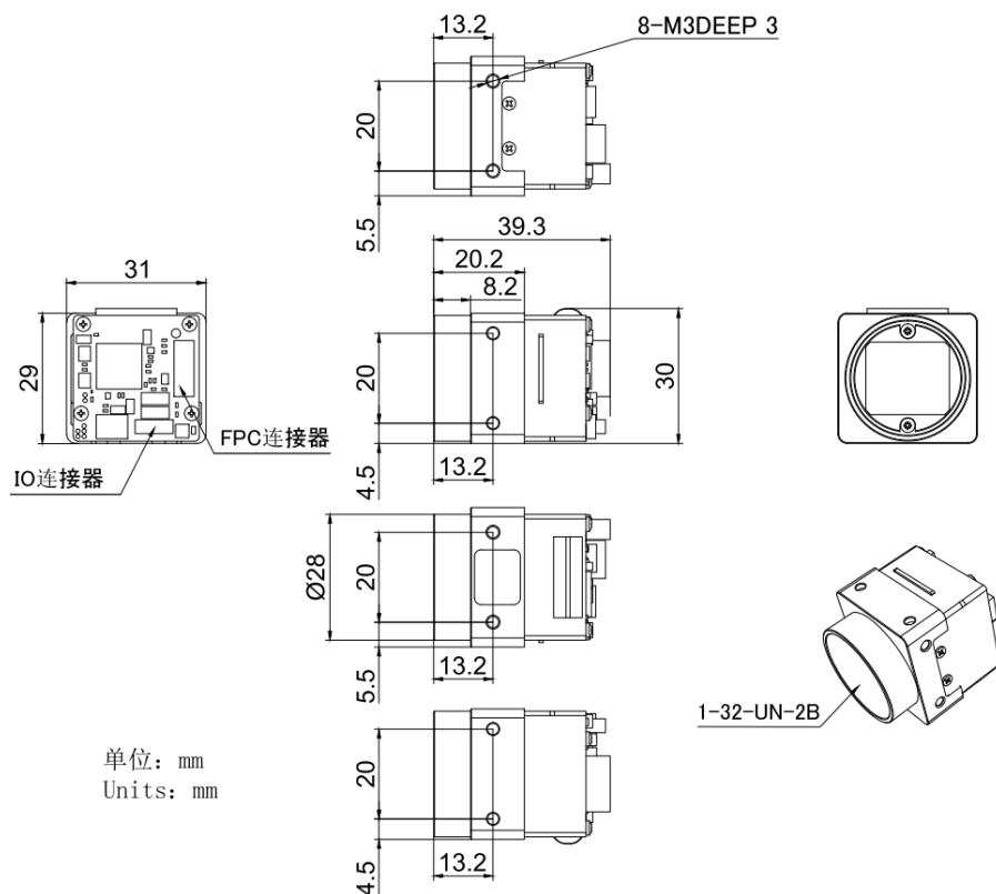
图 5-8 一体式垂直 FPC 相机机械尺寸图
