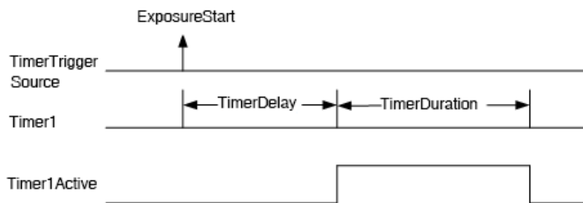
图 8-59 Timer1Active 示意图
