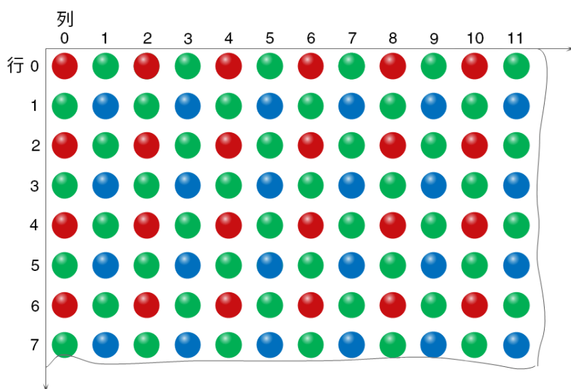
图 8-33 BayerRG8 的像素排列示意图
