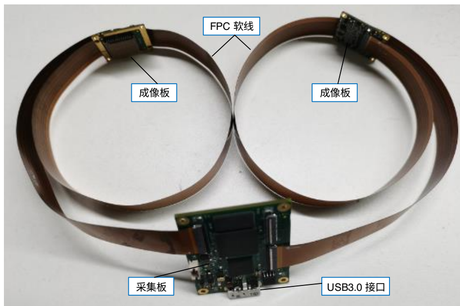
图 3-4 分体式双目相机组成和装配图（无 C-Mount）
