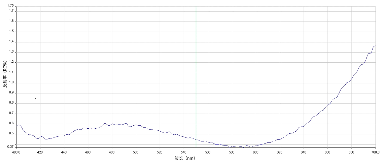
图 6-2 金星 USB3.0 黑白相机透光片反射率曲线
