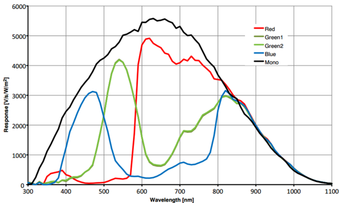
图 4-9 VEN-134-90U3M/C-D SENSOR 响应曲线
