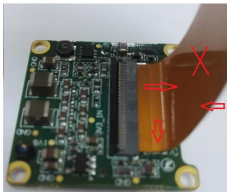
图 3-8 成像板 FPC 线 FPC 座附近禁止外力示意
