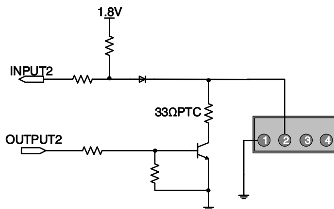
图 7-6 Line2（双向）电路
