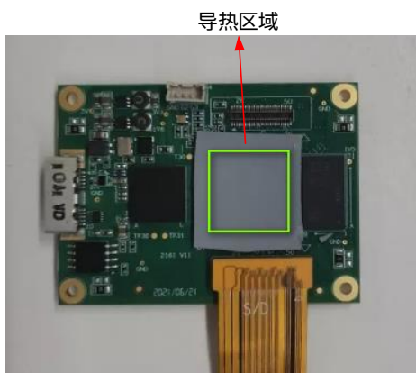
图 3-12 分体式单目相机添加导热材料的区域示意
