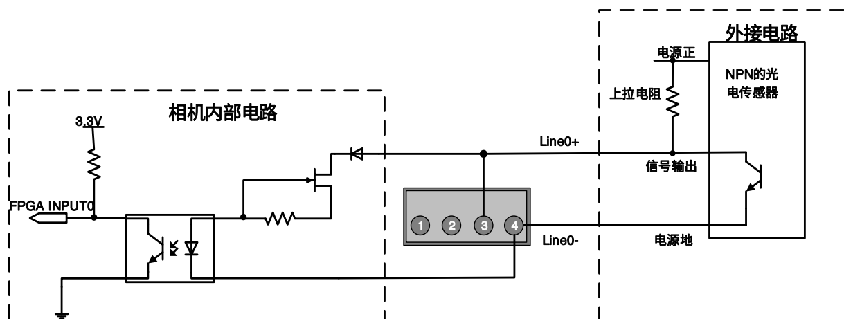
图 7-3 NPN 型光电传感器连接到光耦隔离输入电路
