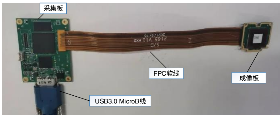
图 3-2 分体式单目相机组成和装配图（无 C-Mount）
