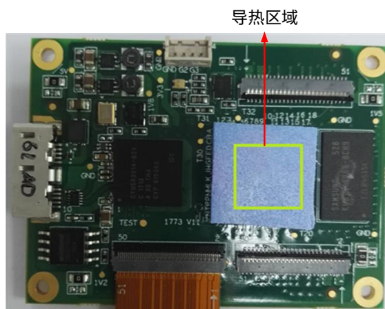
图 3-13 分体式双目相机添加导热材料的区域示意
