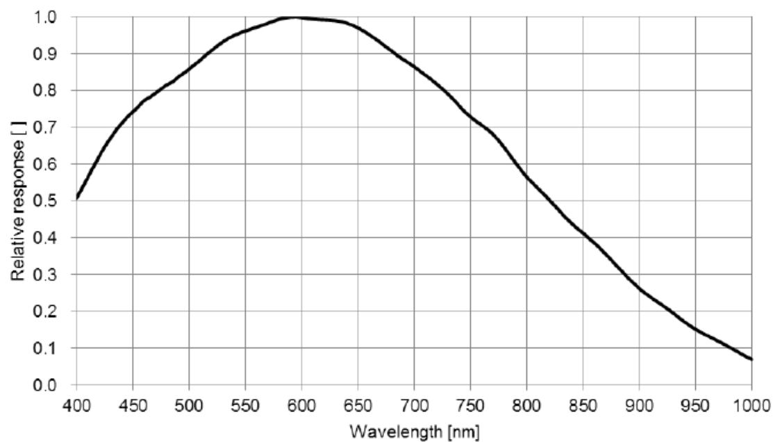
图 4-20 VE2S-301-125U3M-S (J150) SENSOR 响应曲线
